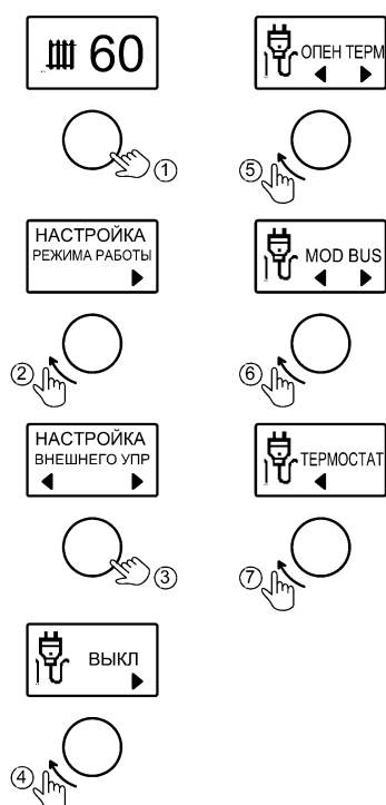
Рисунок 11. Настройка работы от внешнего устройства
