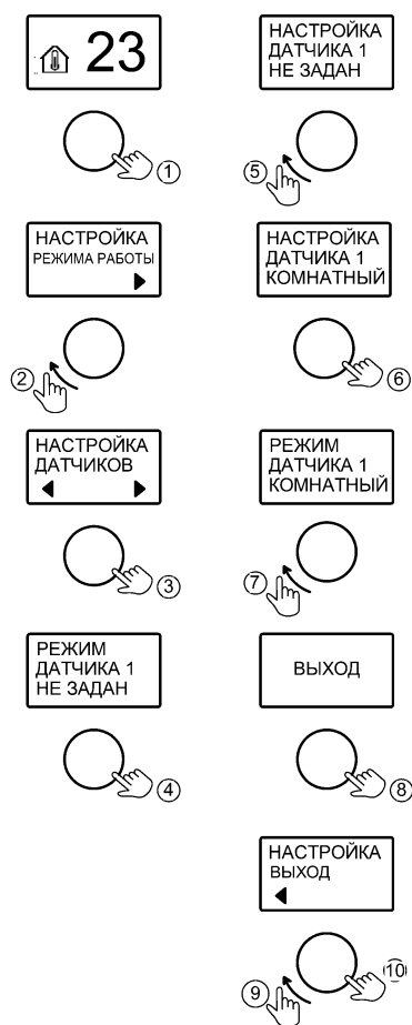
Рисунок 10. Настройка датчиков температуры воздуха
